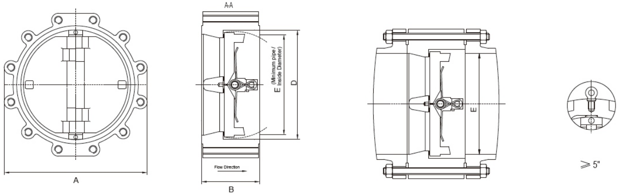
Lug type
