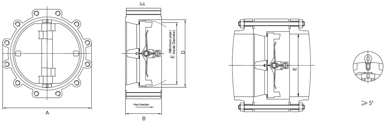
Lug type
